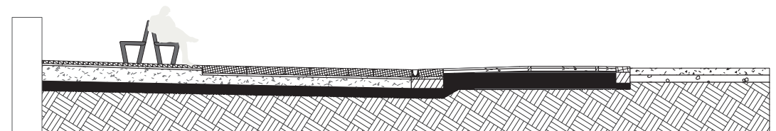
REGELSNITT MESSE SÜD
